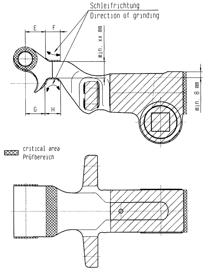
Ilustración 3: Ámbito del ensayo y medidas críticas de la mordaza fija
